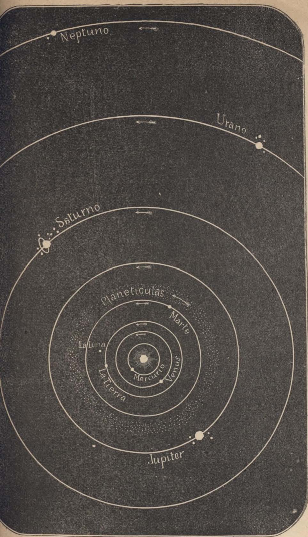
El sistema planetario.
